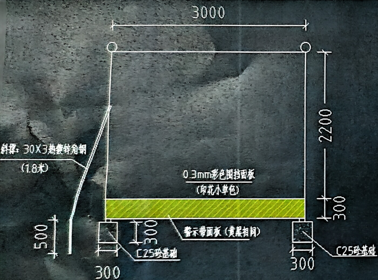
围挡节点大样
