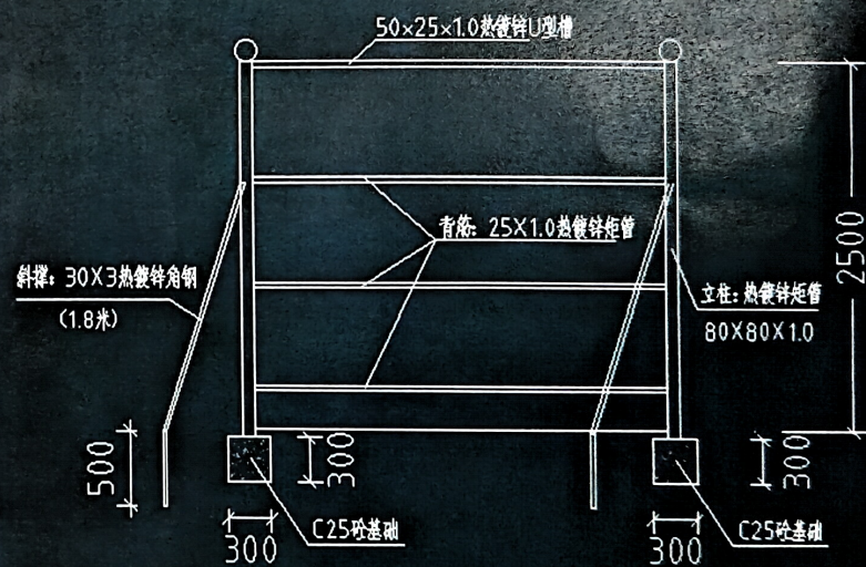
围挡节点大样
